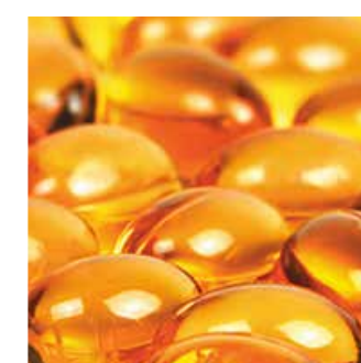
Витамин А
